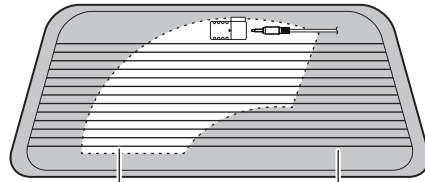
リアワイパー拭き取り (稼働範囲) 熱線
